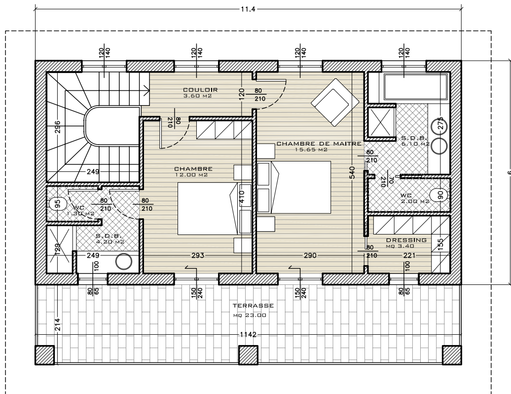
PREMIER ETAGE 1 : 100
